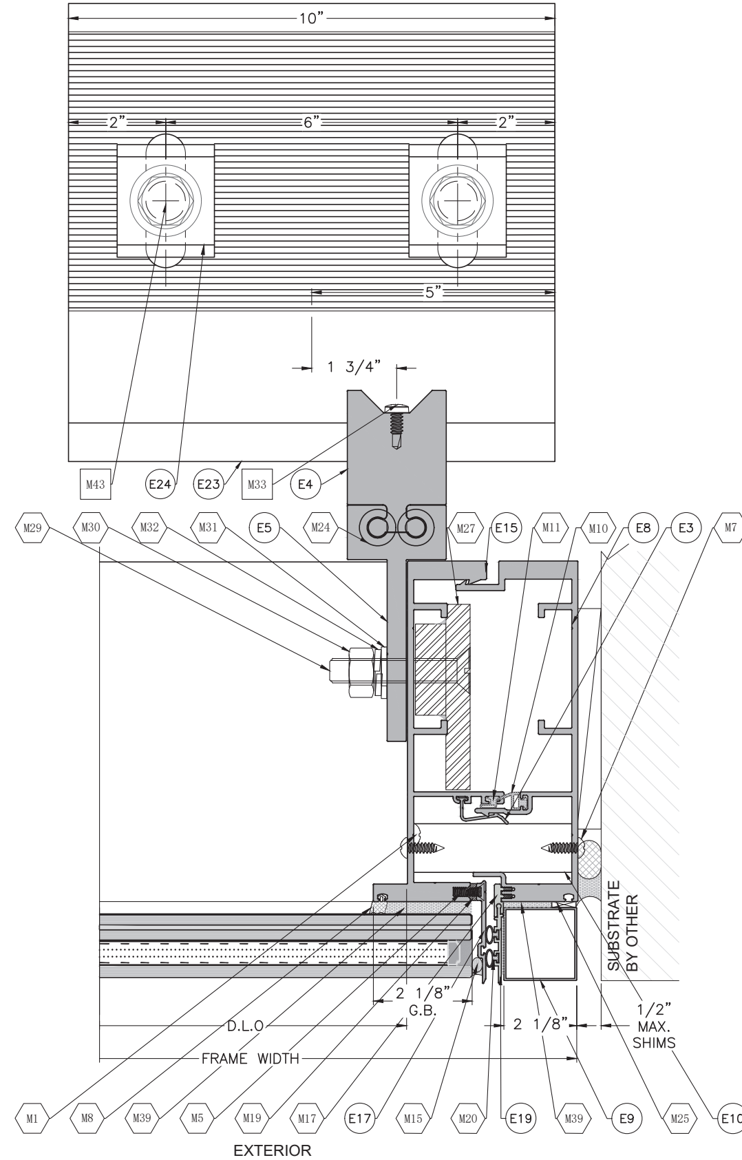
2 D5 DETAIL
