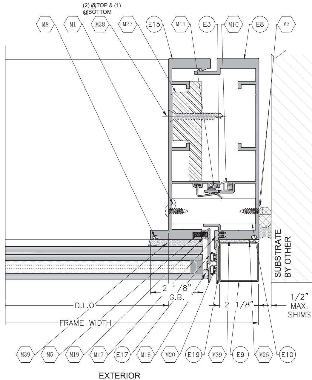
2 D3 DETAIL
