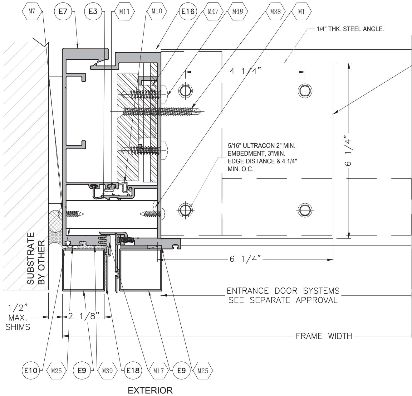
1 D19 DETAIL
