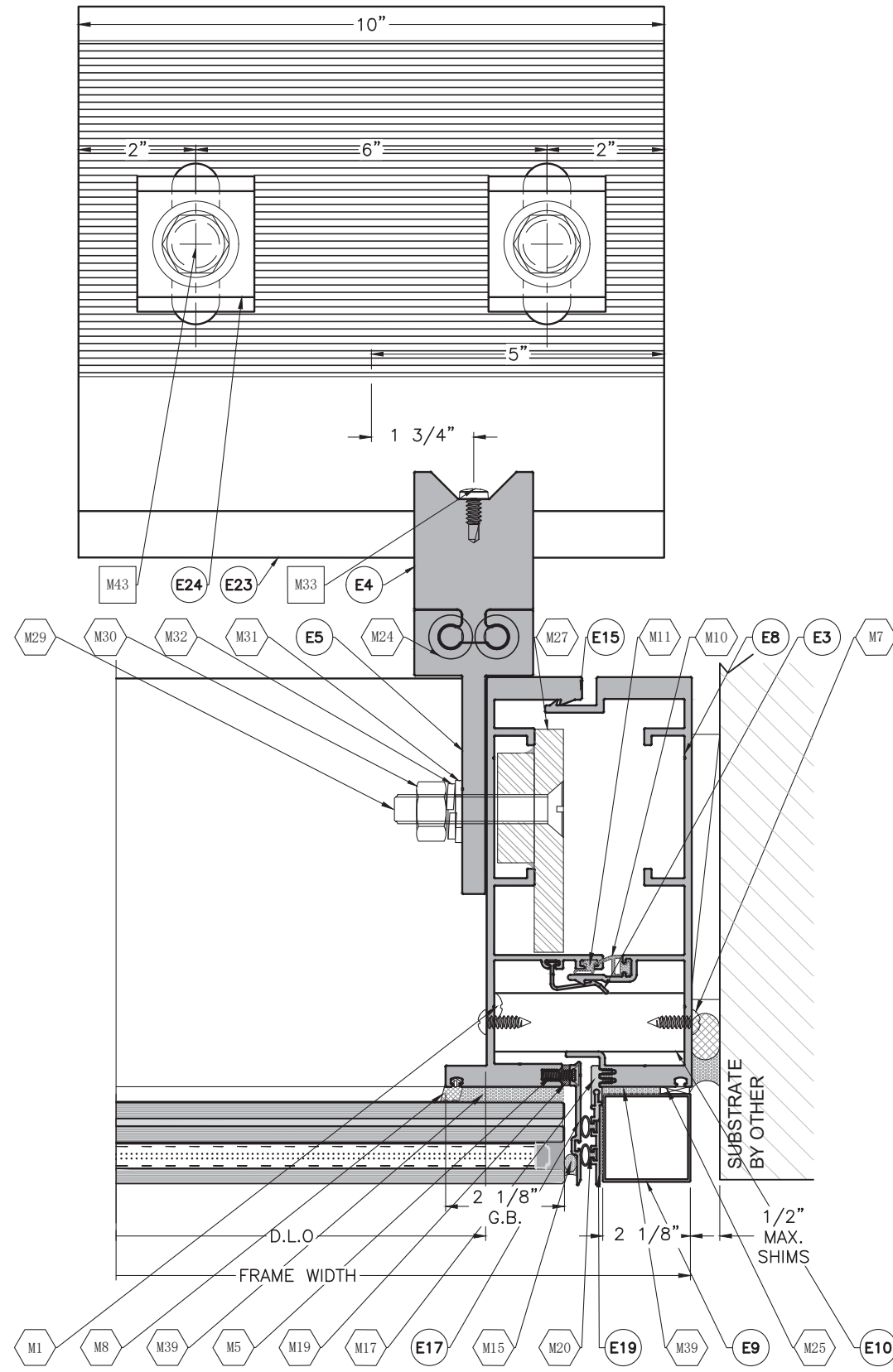
2 D12 DETAIL
