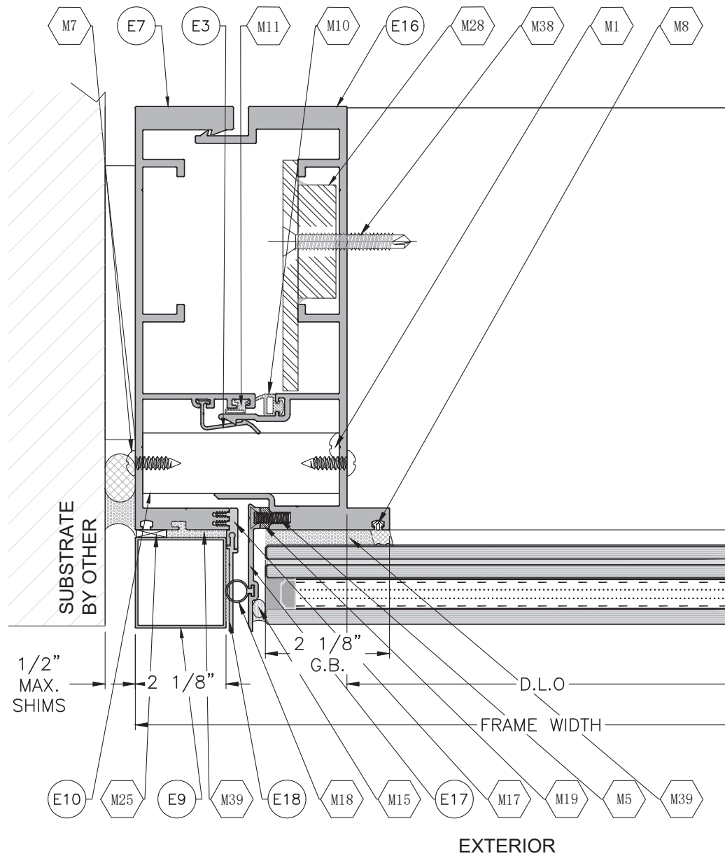
1 D10 DETAIL
