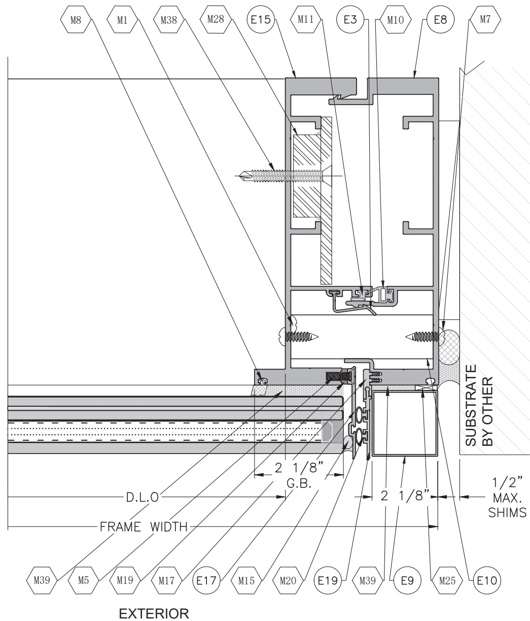
2 D10 DETAIL
