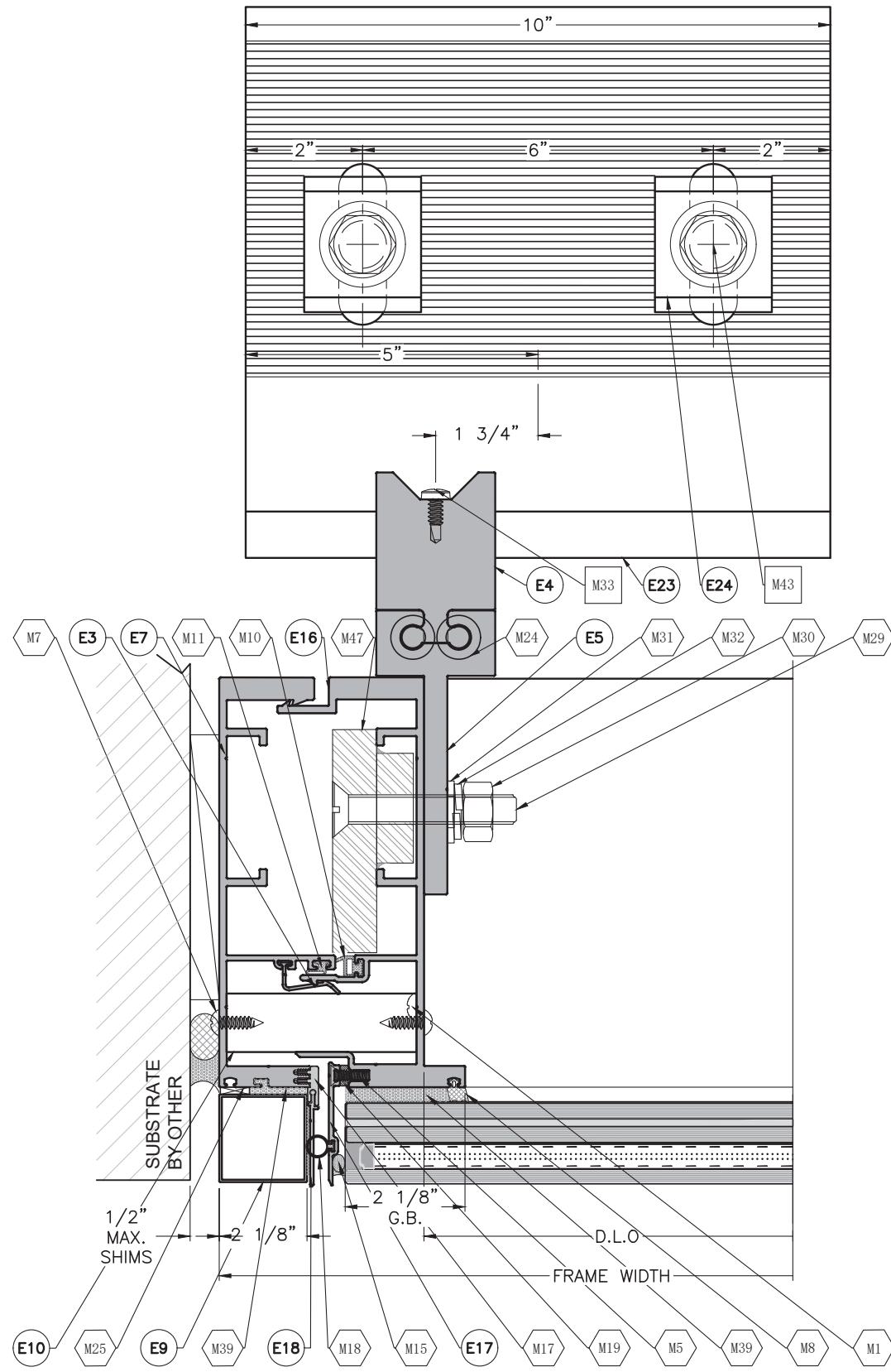
1 D12 DETAIL
